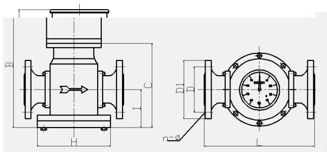
DN65/DN80 (light type)
