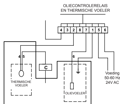
Afb. 10 Aansluiting niveauvoeler
