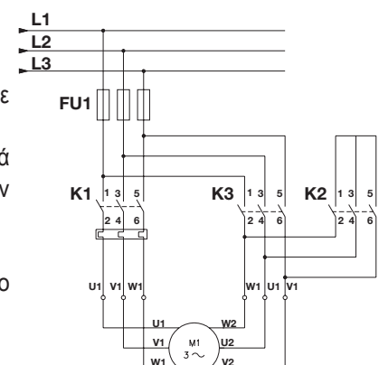
Εικ. 11 Συνδέσεις αστέρα - τριγώνου
