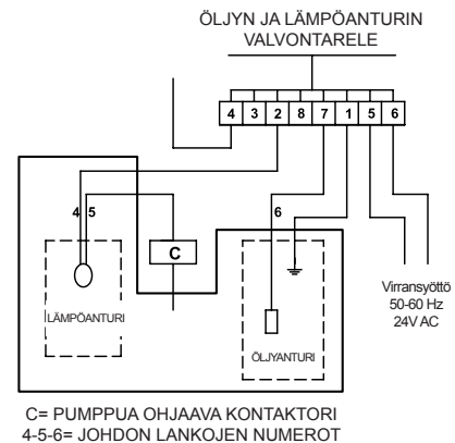
Kuva 13 Lämpöanturin liitäntä
