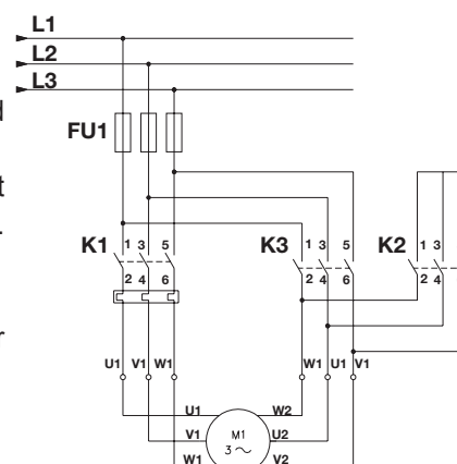
Fig. 11 Stjärn-/triangelanslutningar
