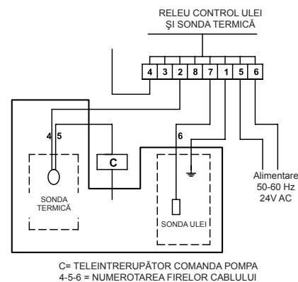
Fig. 13 Conexiune sonda termică
