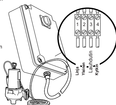
Kuva 9 Sähkötaulu matalajännitte pumpuille
