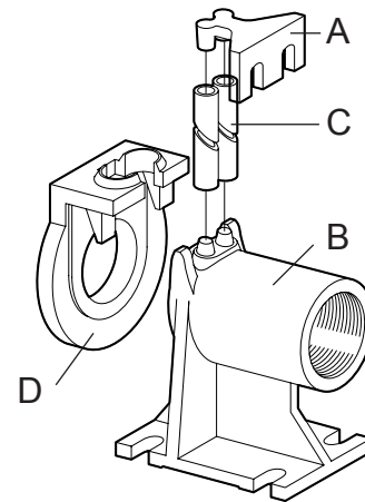
Kuva 7 Kytcentäjalka
