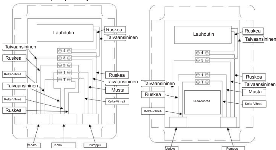
Kuva 9 Sähkötaulu matalajännitte pumpuille
