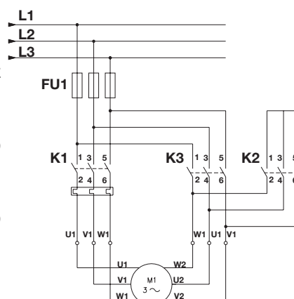
11. ábra: Csillag-delta bekötés
