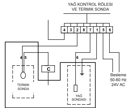
C= POMPA KUMANDA TELERÜPTÖRÜ 4-5-6 = KABLOLUN TELLERİ NUMARALANDIRILMASI
