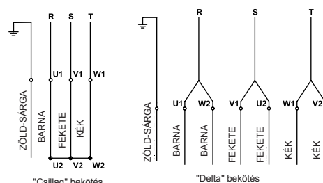
10. ábra: háromfázisú bekötés direkt indításhoz
