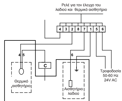
Εικ. 13 Σύνδεση θερμικού αισθητηρίου
