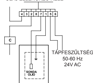
14.ábra: az olajszonda bekötése
