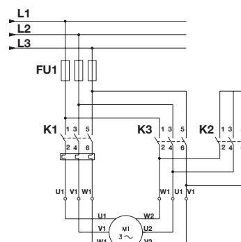
Afb. 11 Ster-driehoekaansluitingen
