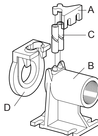
Obr. 7 Spojovací noha
