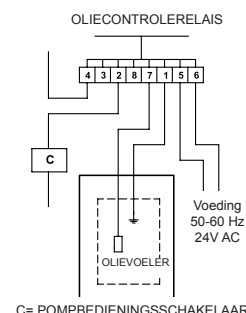
Afb. 11 Aansluiting niveauvoeler
