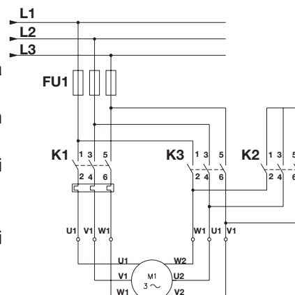
Kuva 11 Tähti-kolmio liitännät
