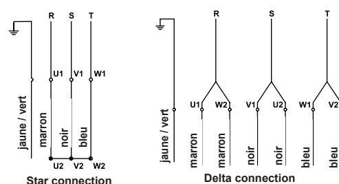
Fig. 10 branchement triphasé pour démarrage direct
