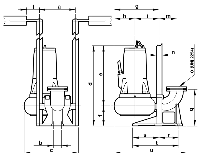
Fig. 18 Series FEKA 3000 - FEKA RC 3000 FEKA 4000 - FEKA 6000 - FEKA 8000
