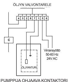
Kuva 14 Tasoanturin liitäntä
