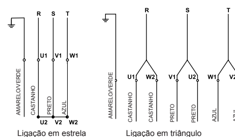
Fig. 10 Ligações trifásicas para arranque directo
