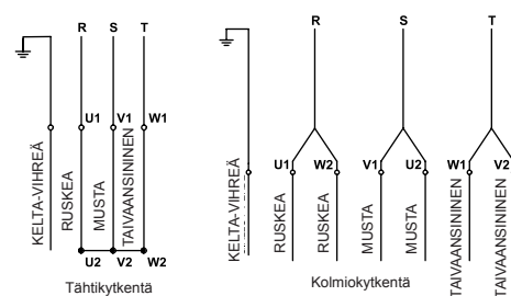
Kuva 10 Kolmivaiheiliitännät suoraa käynnistystä varten
