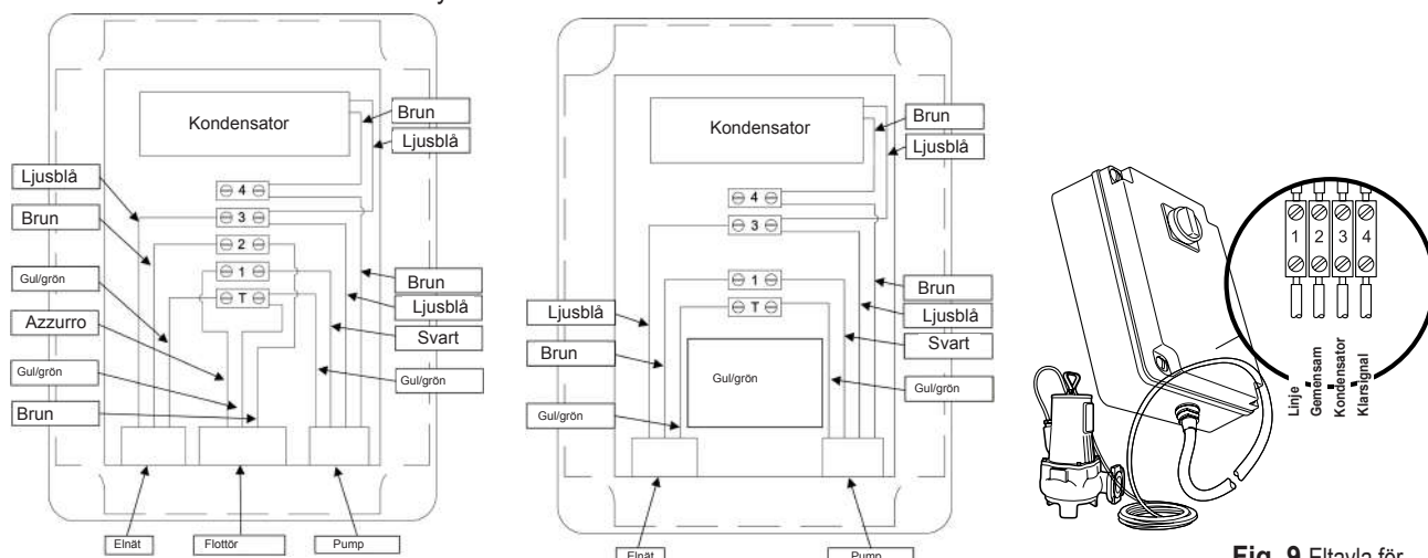
Fig. 9 Eltavla för lågspäningspumpar
