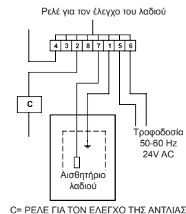
Εικ. 14 Σύνδεση αισθητηρίου στάθμης!
