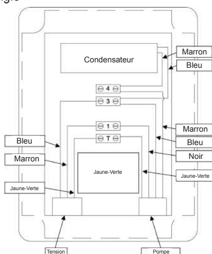
Fig. 8 Schémas de branchement électrique avec et sans interrupteur automatique à flotteur.
