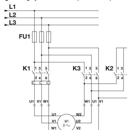
Fig. 11 Ligações estrela triângulo
