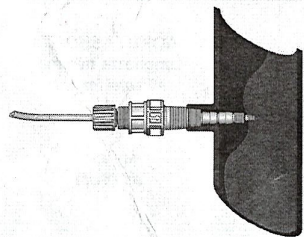
INSTALLAZIONE SU ATTACCO 3/8" INSTALLATION SU ATTACCO 3/8"
