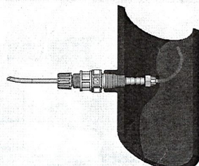
INSTALLAZIONE SU ATTACCO 1/2" CON PROLUNGA FLESSIBILE 4x6 ANTI INCROSTAZIONI / INSTALLATION ON 1/2" CONNECTION WITH ANTIFOAM 4x6 FLEXIBLE EXTENSION
